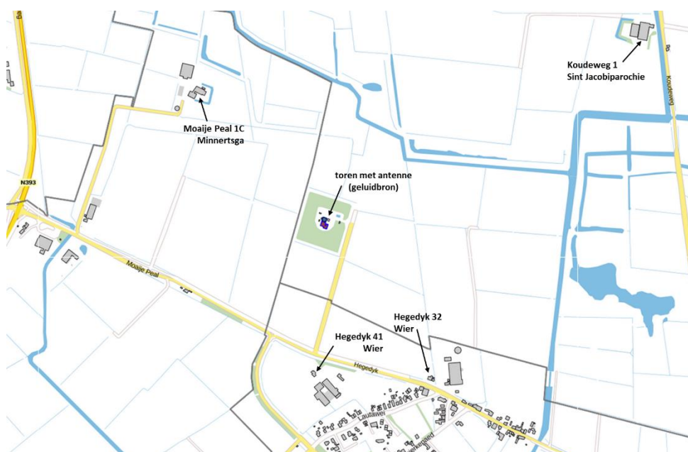
Figuur 2: Beoogde locatie van de toren met radarantenne en de dichtstbijzijnde geluidgevoelige bestemmingen (woningen) in de gemeente Waadhoeke (Friesland).
